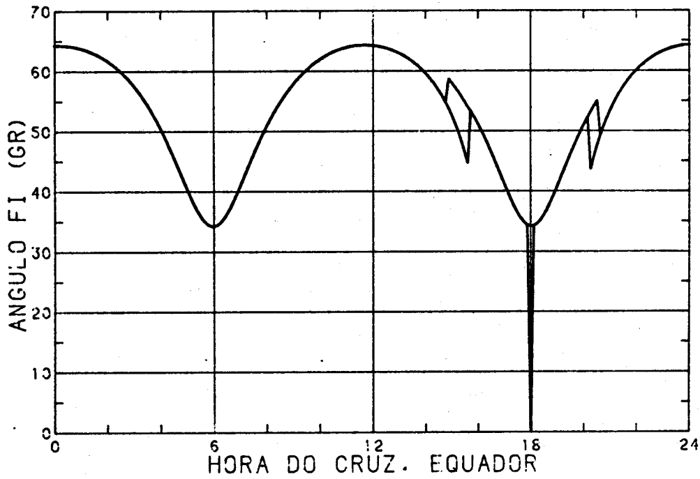
Fig. 4.3 - Ângulo \phi_0 em função do horário de cruzamento, \bar{h} .
