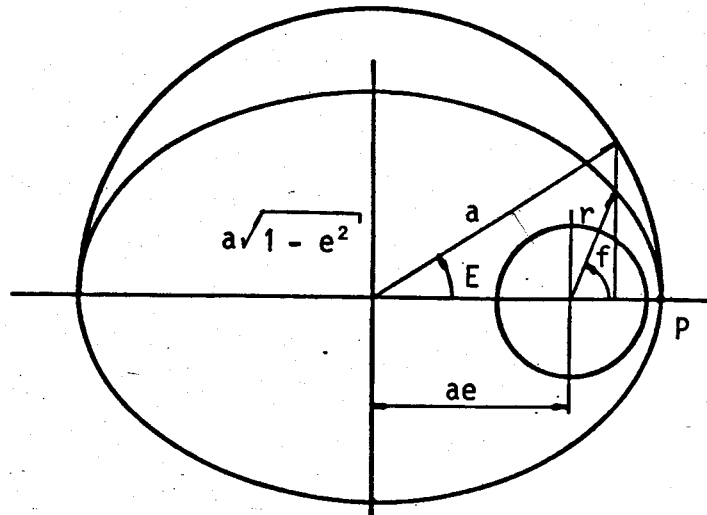
Fig. 2.2 - Elipse orbital.
