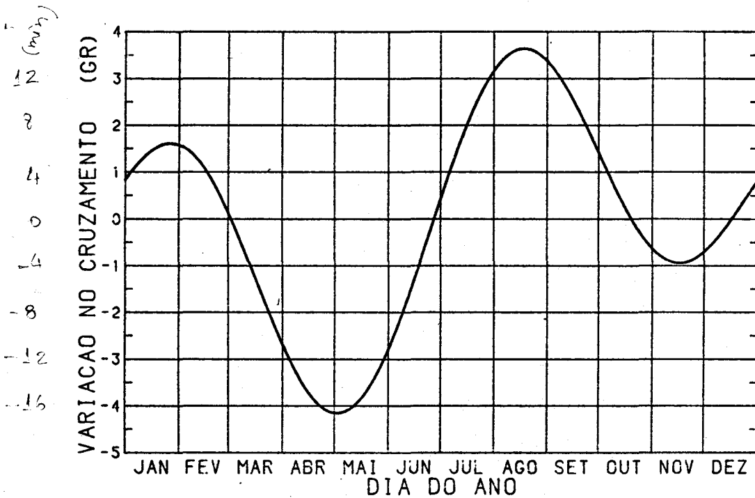
Fig. 2.6 - Variação no horário de cruzamento com equador em um ano.
