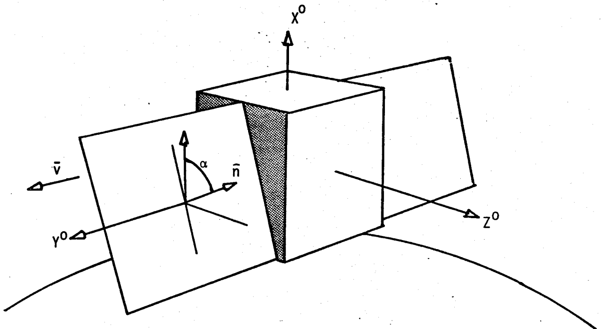
Fig. 3.2 - Sistemas X^0Y^0Z^0 e X^uY^uZ^u .
