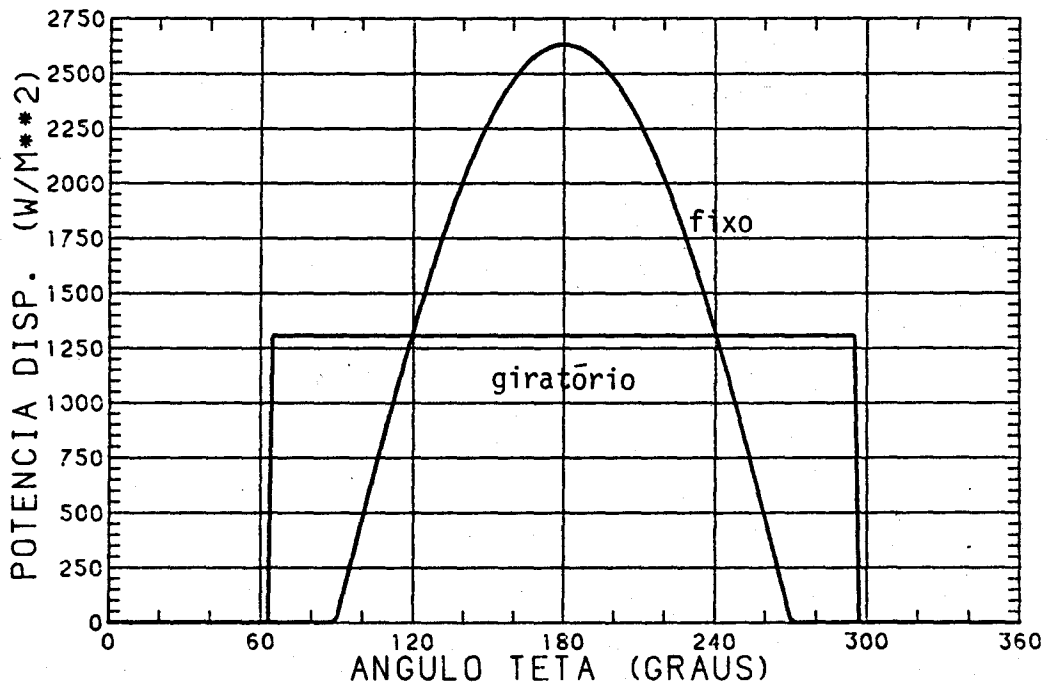
Fig. 5.5 - Potência disponível ao longo de uma órbita para h = 12:00 h. Energia na órbita igual para ambos os tipos de painéis.
