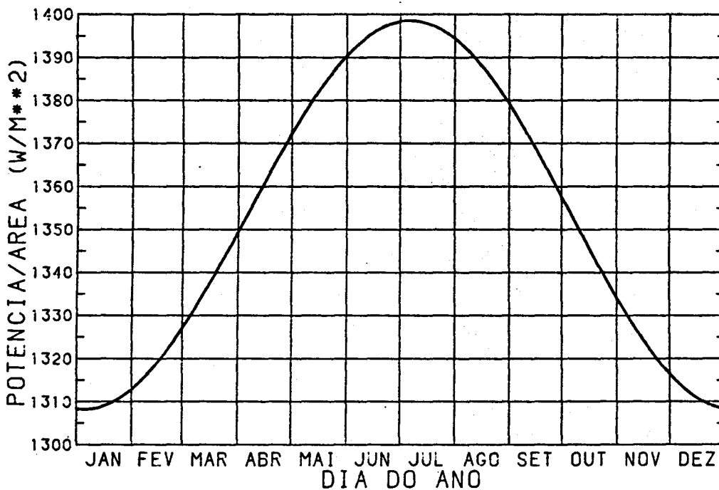
Fig. 2.8 - Variação na potência por unidade de área incidente num painel perpendicular aos raios solares, em função da época do ano.
