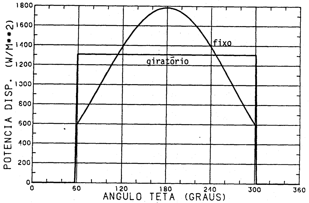
Fig. 5.4 - Potência disponível ao longo de uma órbita para o horário de cruzamento h = 9:00 h. Energia disponível na órbita igual para ambos os painéis (áreas diferentes).
