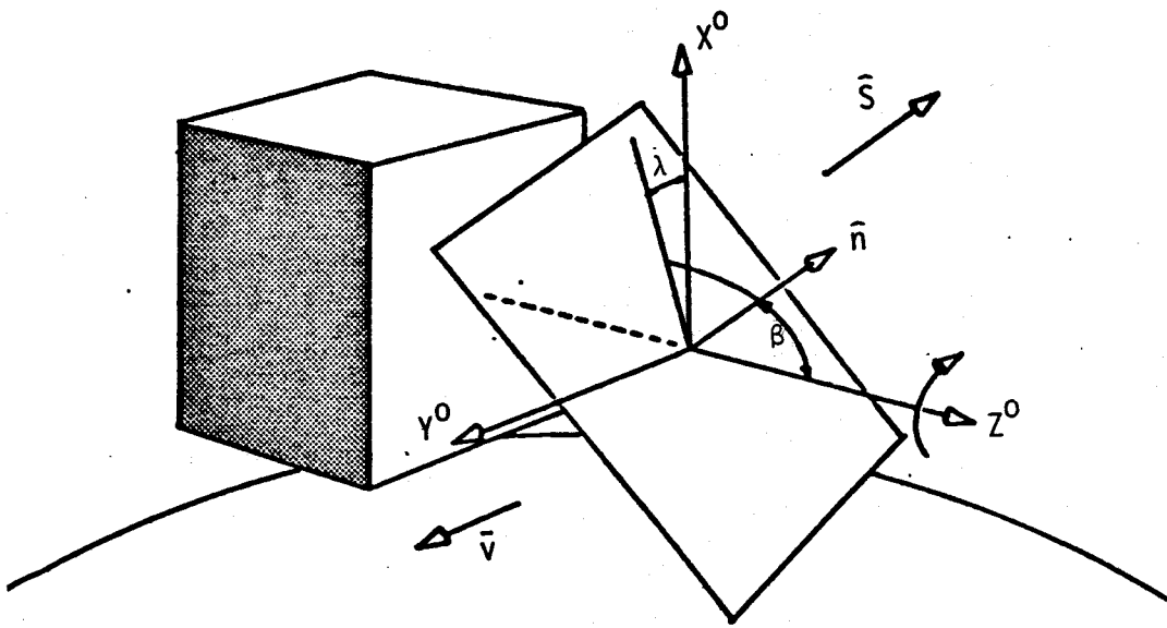
Fig. 4.1 - Satélite com painéis giratórios.
