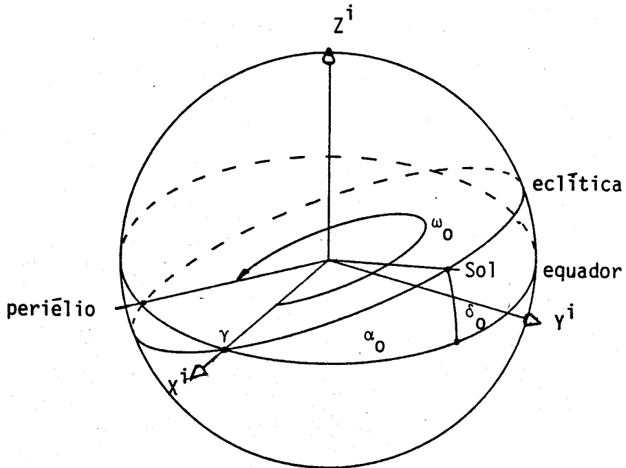
Fig. 2.3 - Ascensão reta, \alpha_0 , e declinação, \delta_0 , do Sol.
