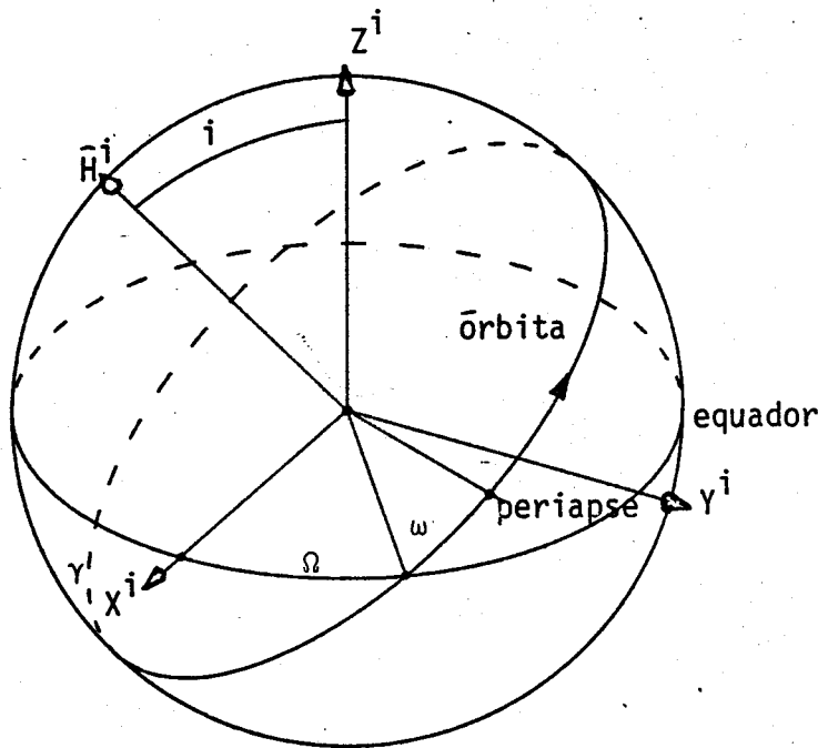
Fig. 2.1 - Elementos orbitais angulares.
